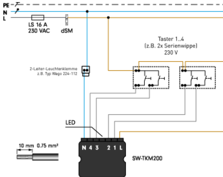
Abb. 14: Montageanleitung für die digitalSTROM-Tasterklemme SW-TKM200
