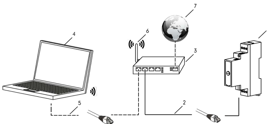
Abb. 19: Verbinden des digitalSTROM-Systems mit dem Netzwerk LAN. digitalSTROM-Server (1), RJ45-Netzwerkkabel (2, 5), DHCP-fähiger Netzwerk-Router (3), Laptop (4), drahtloses Netzwerk WLAN (6)
