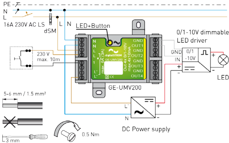
Abb. 10: Montageanleitung des digitalSTROM-UMV (GE-UMV200)
