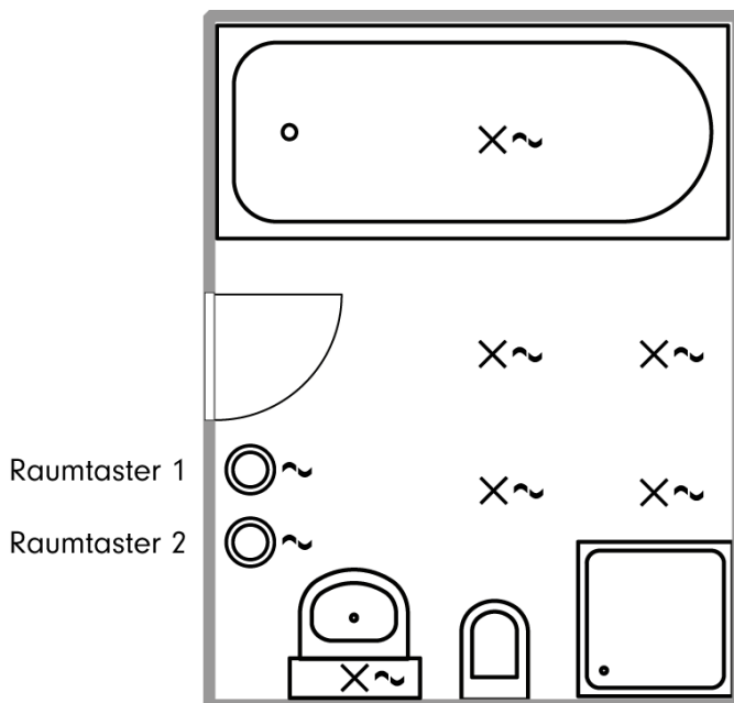
Abb. 51: Raumplan Badezimmer mit zwei Raumtastern
