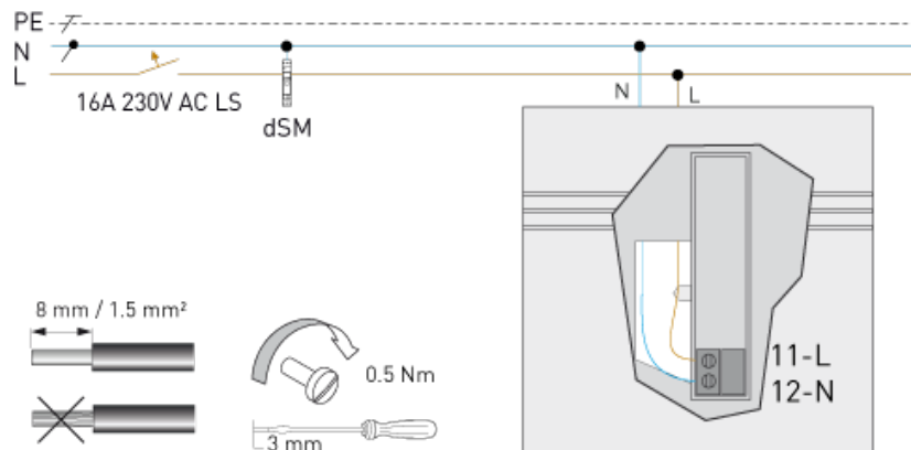
Abb. 17: Montageanleitung des digitalSTROM-Raumklima-Sensors dS-iSens200
