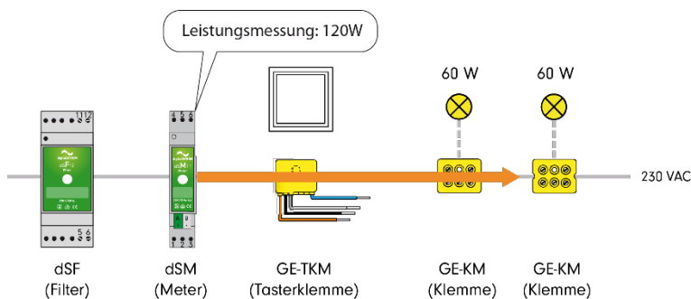
Abb. 3: Beispiel für eine digitalSTROM-Installation, Hinkanal
