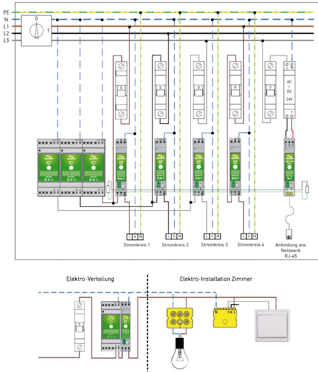
Abb. 1: digitalSTROM-System Grundschemata Elektroverteilung
