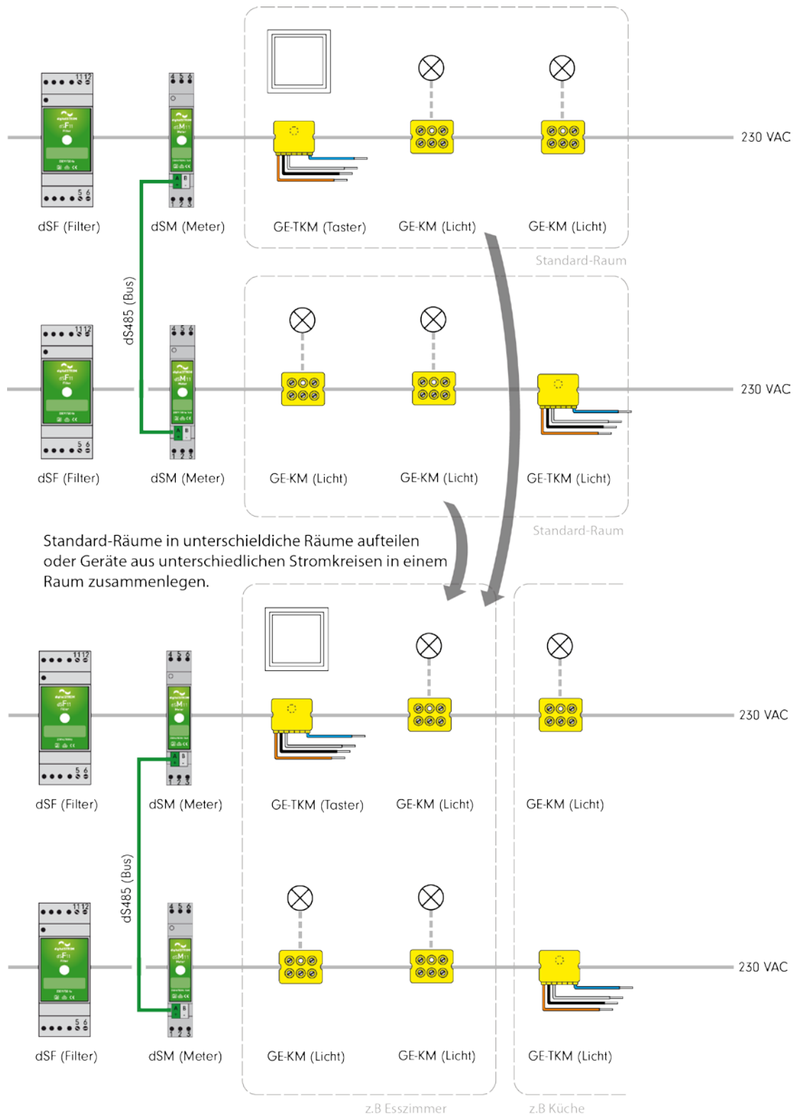
Abb. 47: digitalSTROM-Installation mit digitalSTROM-Geräten an vier digitalSTROM-Metern
