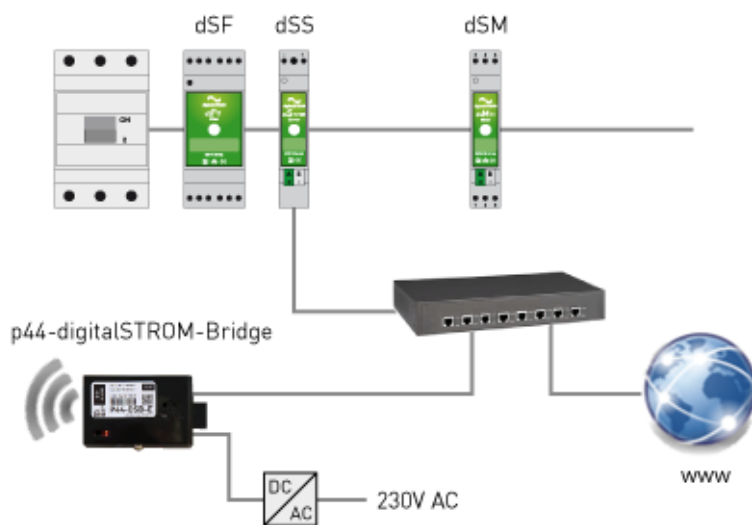
Abb. 7: Montage von funkbetriebenen Geräten via Plan44-Bridge im digitalSTROM-System
