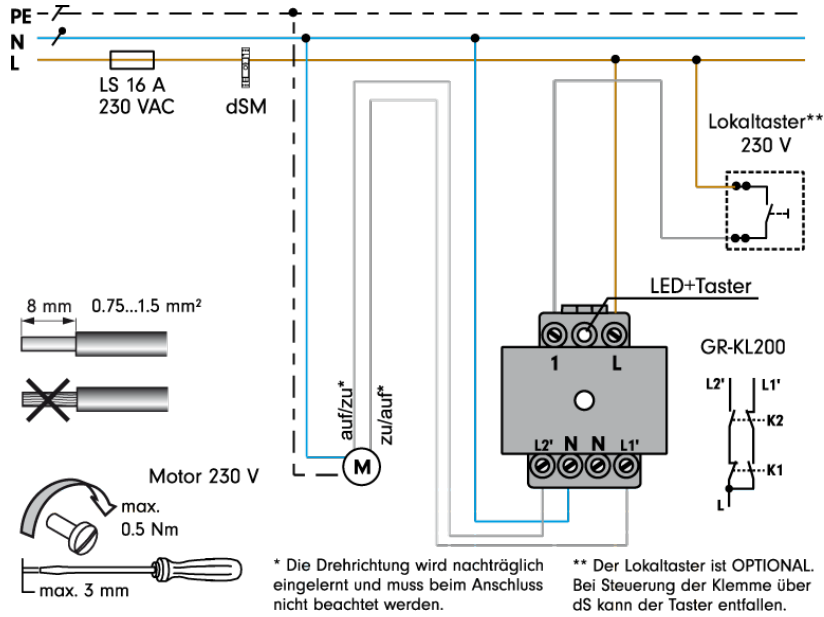
Abb. 11: Montageanleitung der digitalSTROM-Relaisklemme GR-KL200
