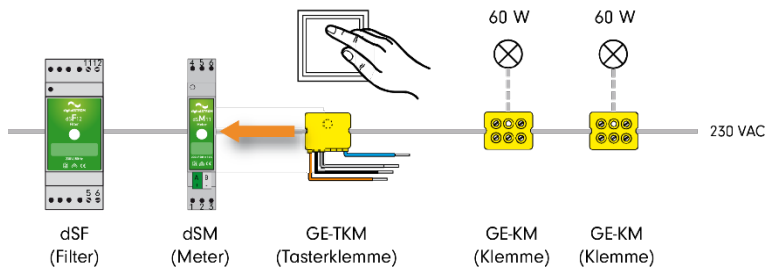
Abb. 2: Beispiel für eine einfache digitalSTROM-Installation, Rückkanal
