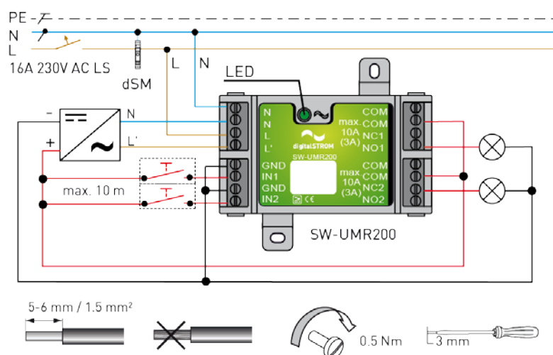
Abb. 15: Montageanleitung für das digitalSTROM SW-UMR200
