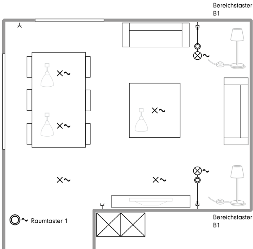
Abb. 49: Raumplan Wohnzimmer mit einem Raumtaster und zwei Bereichstastern
