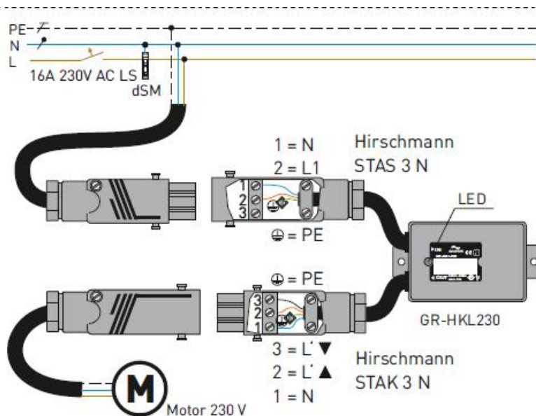
Abb. 12: Montageanleitung für den digitalSTROM-Jalousie-Schaltaktor GR-HKL230
