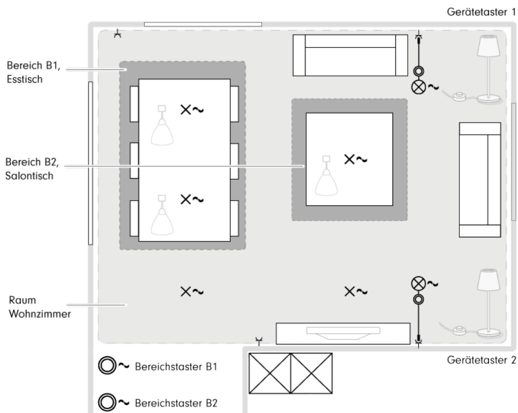
Abb. 48: Beispiel für die Einteilung eines Raumes in verschiedene Bereiche
