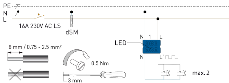
Abb. 16: Montageanleitung für die digitalSTROM-Klimaklemme BL-KM200
